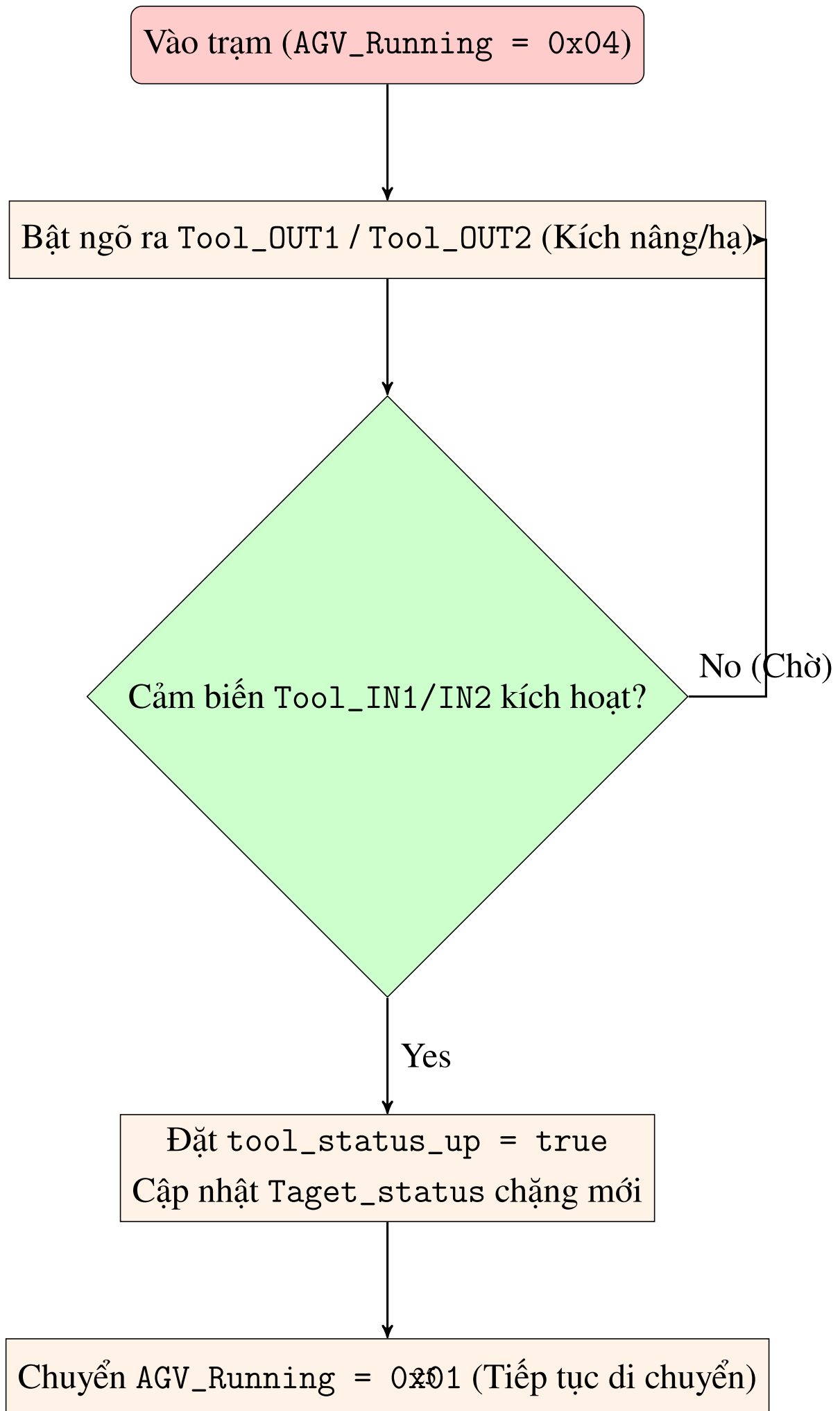
Hình 3.8 Sơ đồ tuần tự quy trình nâng/hạ móc kéo hàng tự động.
