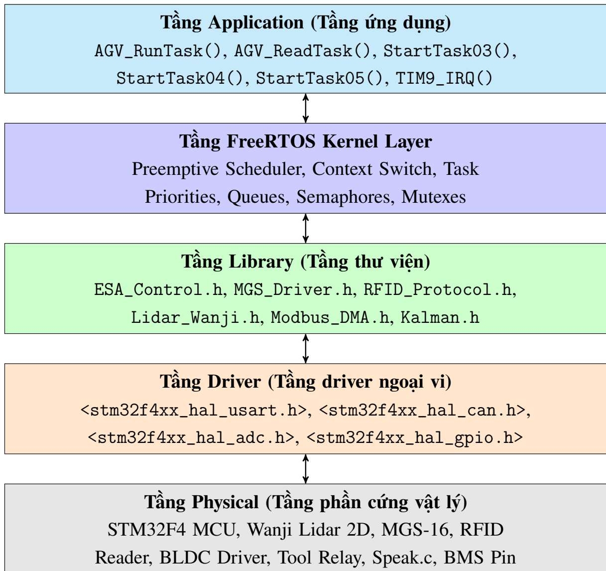
Hình 3.4 Sơ đồ kiến trúc phần mềm nhúng STM32F4.
