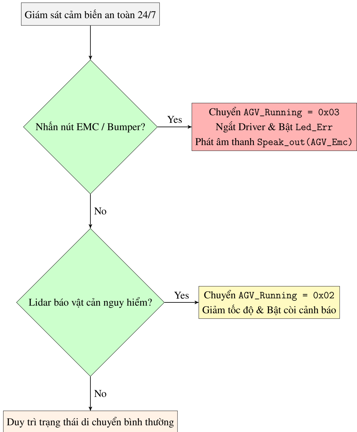
Hình 3.7 Sơ đồ tuần tự xử lý an toàn Lidar, Bumper và Nút khẩn cấp.
